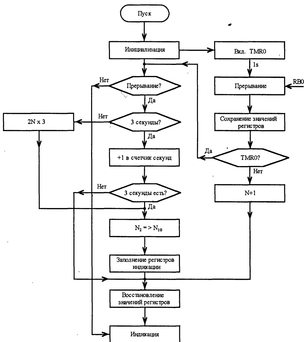
Алгоритм функционирования электронного устройства
